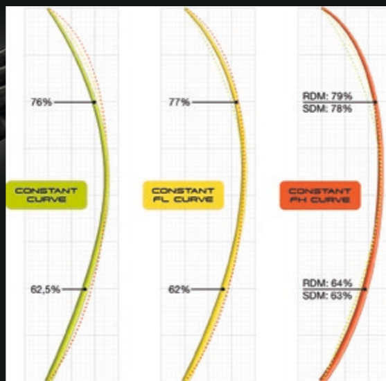
Srovnání ohybových charakteristik Constant Curve, Constant FL a Constant FH
